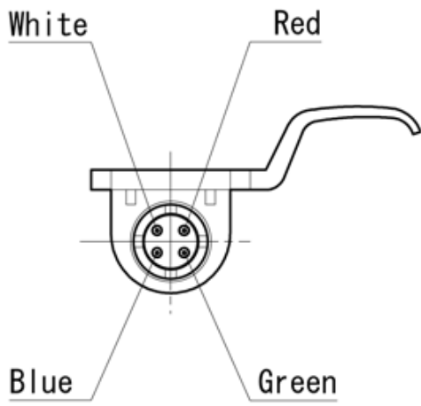
Zeichnung TK 50
